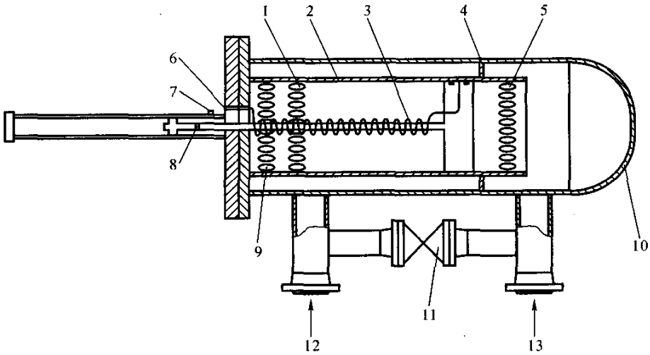
图 4 带外旁通阀的单向活塞体积管
