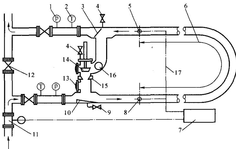
图 1 单向型体积管
