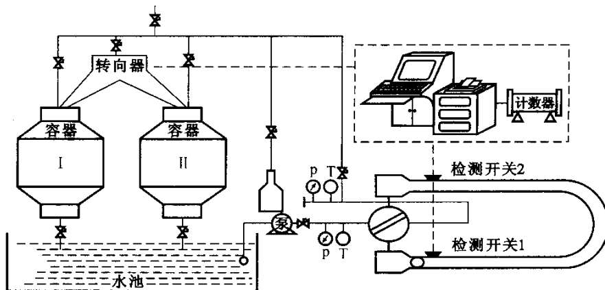
图 6 容积法体积管检定装置
