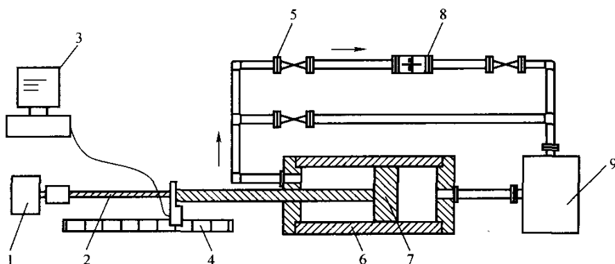
图 5 主动式活塞体积管
