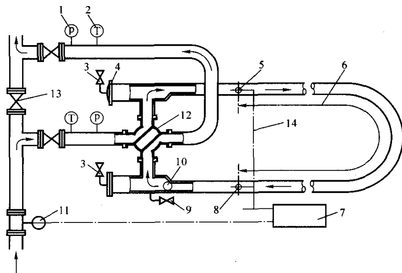
图 2 双向型体积管
