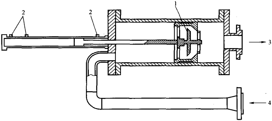
图 3 带内提升阀的单向活塞体积管
